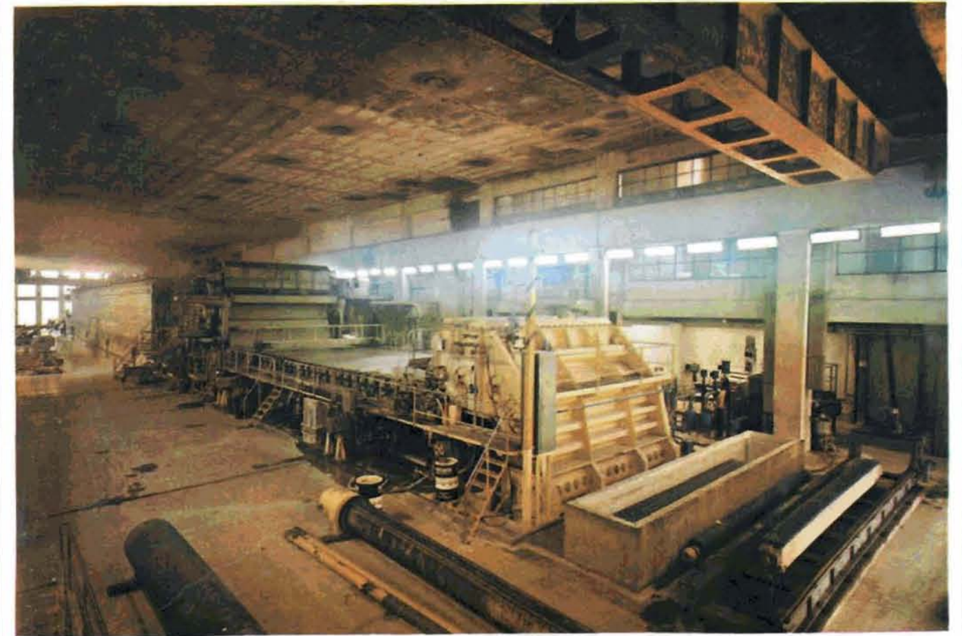
Vista de la nave donde está situada la máquina número V de papel prensa (220 Tm. diarias), de LA PAPELERA ESPAÑOLA, S. A., en Rentería (Guipúzcoa)
