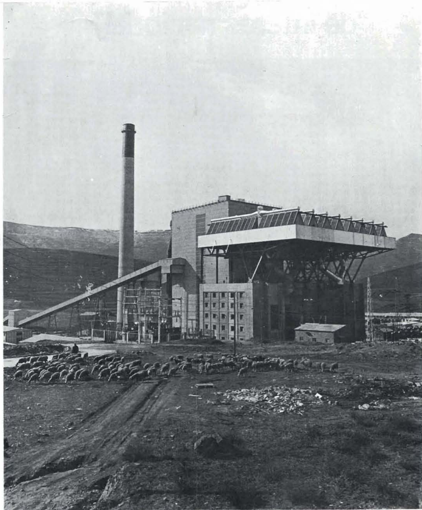
CENTRAL TERMICA DE UTRILLAS.—En la fotografía, una vista parcial de esta central. Construida y explotada por una sociedad en la cual Fuerzas Eléctricas de Cataluña, S. A., tiene una importante participación
